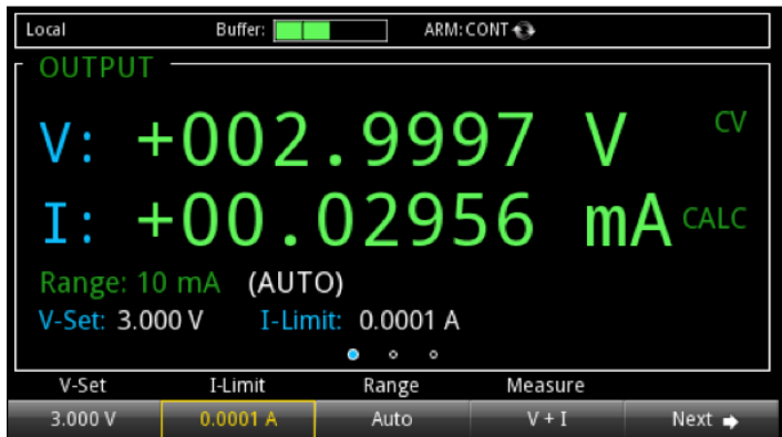
图10. 利用2280S系列电源对高精度基准电压源待测器件进行低电流测量
