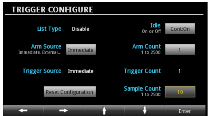
图8. 进行低电流测量时2280S系列电源触发器设置
