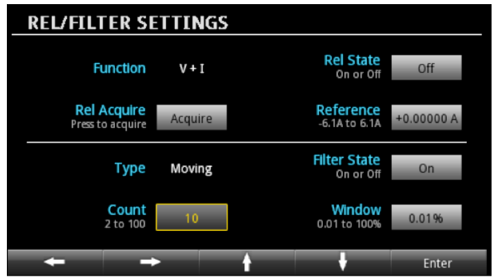
图7. 进行低电流测量时2280S系列电源滤波器的设置
