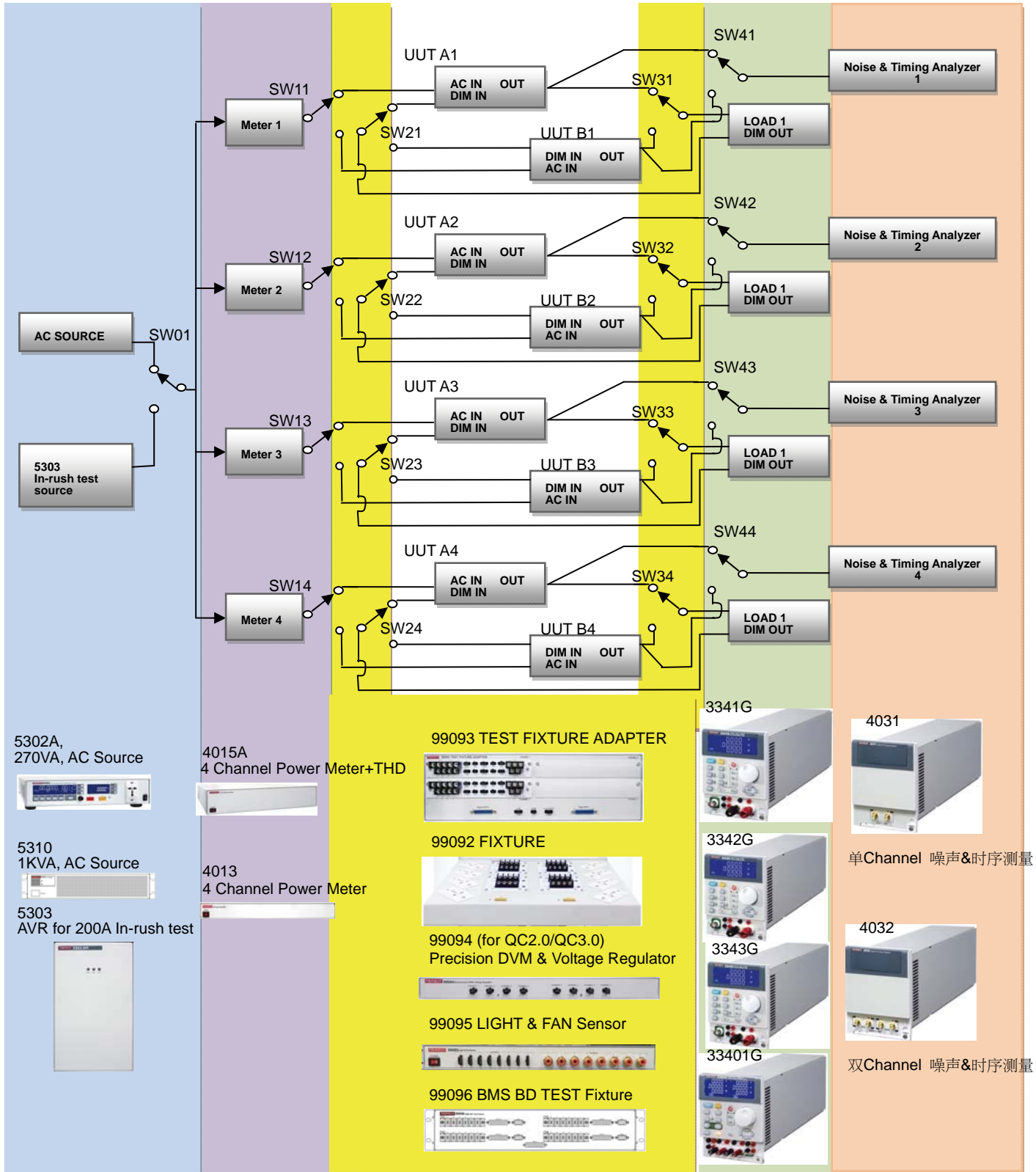
6010 ATE 的系统架构图
