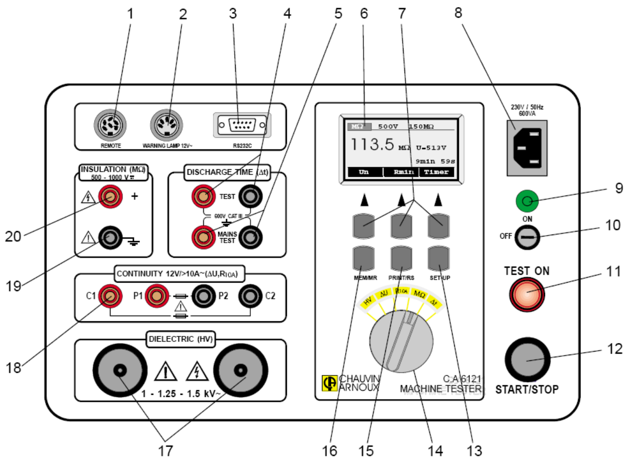
图 1. 前面板外观
