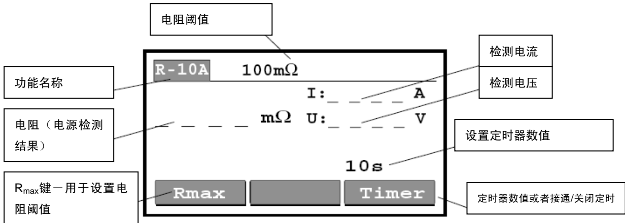
图 12. 位置R 10A 处的主屏幕
