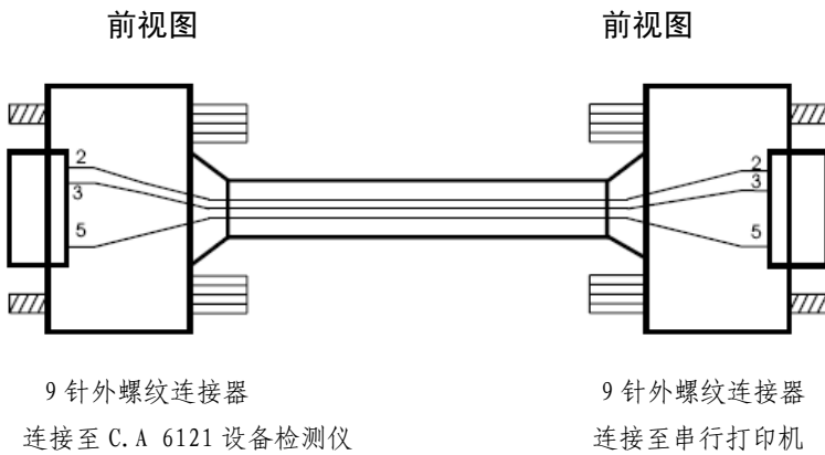
图 29. RS232 通信电缆（打印机）
