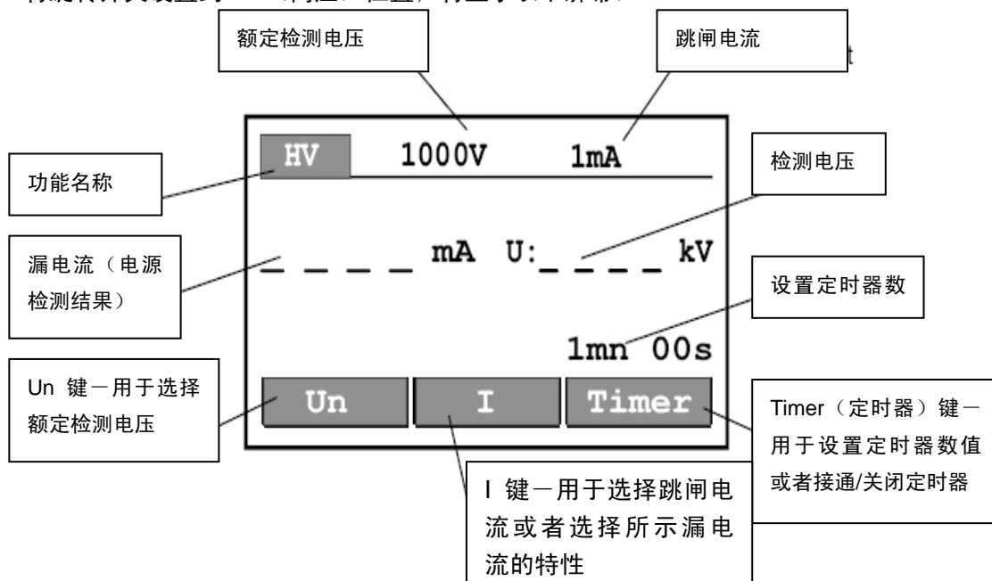
图 4. HV 位置处的主屏幕
