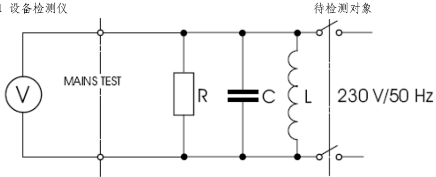
图 19. 检测电路
