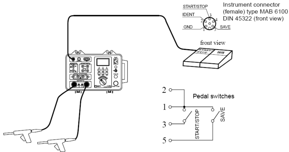
图 41. 遥控踏板与 C.A 6121 设备检测仪的连接
