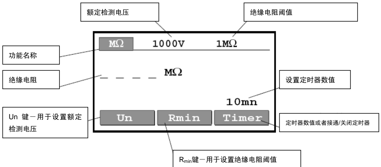
图 16. MW 位置处的主屏幕
