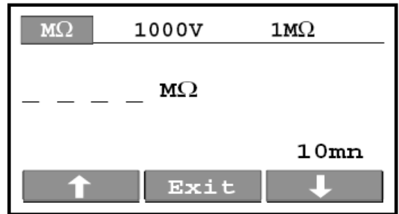
图 17. 绝缘电阻阈值选择菜单
