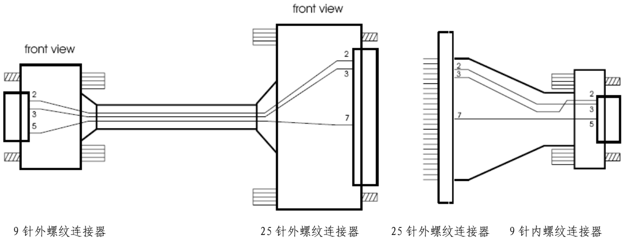
图 31. RS232 通信电缆（个人计算机）和 25—9 针适配器
