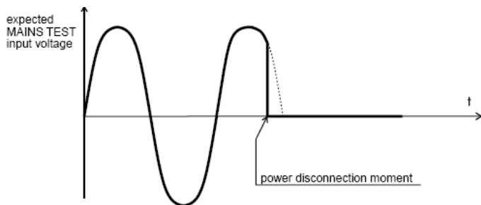
图 24. 电源检测输入上的预期电压
