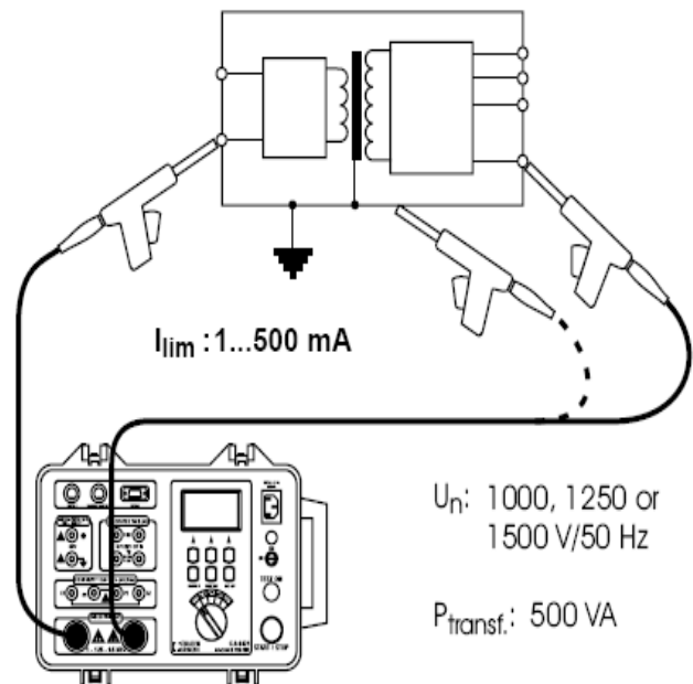
图 8. 检测探针的连接
