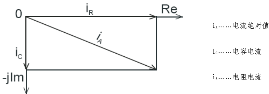
图 3. 检测电流图
