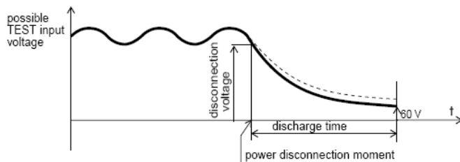
图 25. 检测输入上的预期电压
