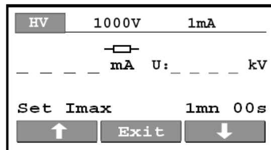
图 6. 跳闸电流选择菜单
