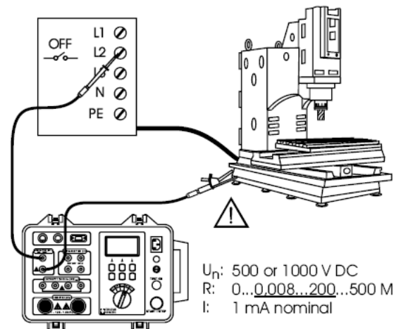
图 18. 检测线的连接
