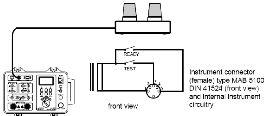
图 43. 警告灯与 C.A 6121 设备检测仪的连接
