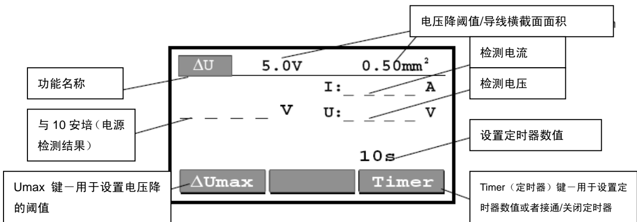
图 10. DU（电压降）位置处的主屏幕
