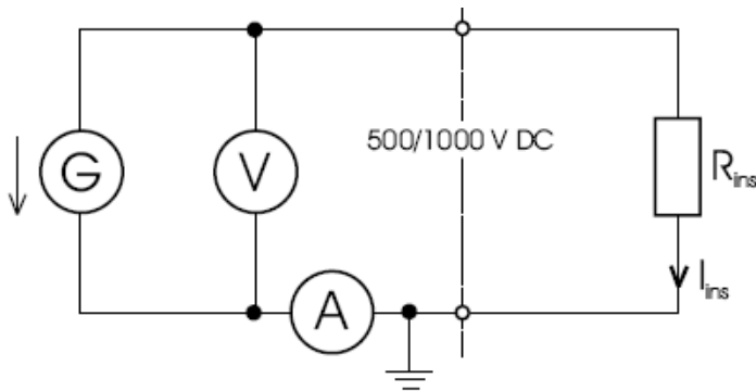
图 15. 检测电路
