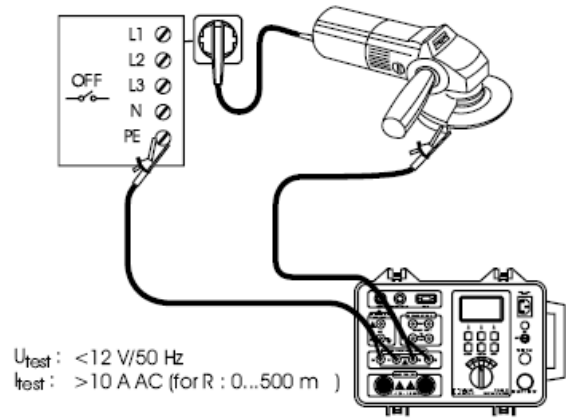
图 14. 检测线的连接
