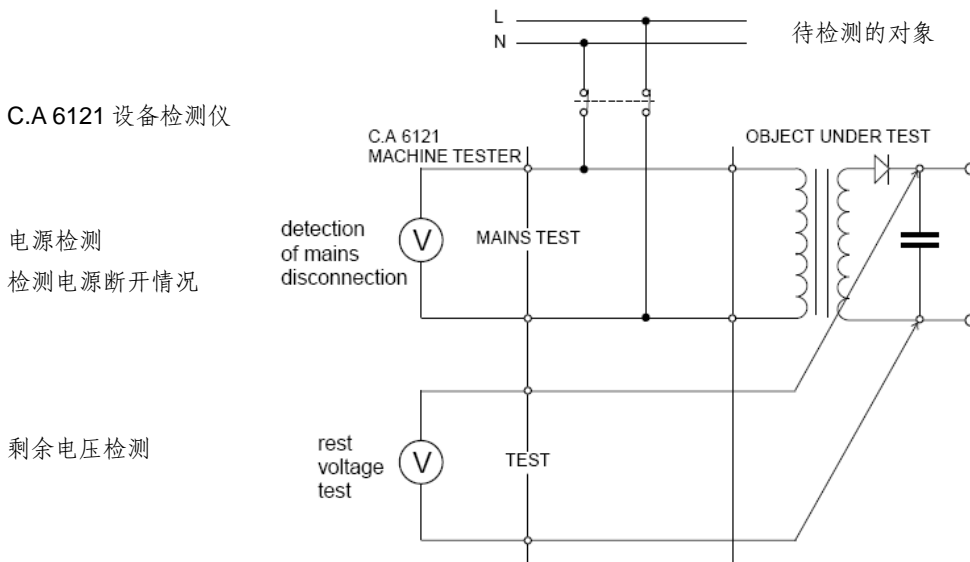
图 23. 检测电路
