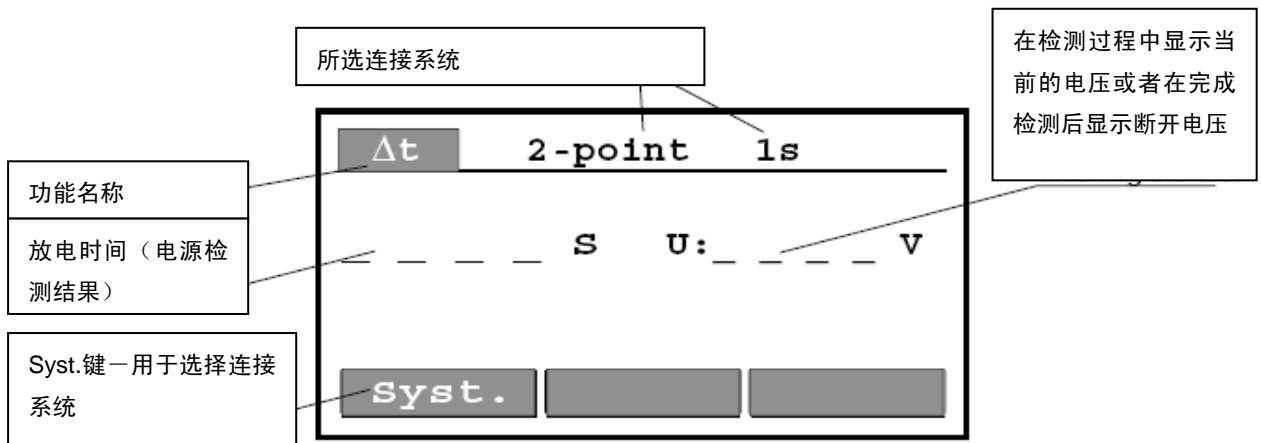
图 21. Dt 位置处的主屏幕
