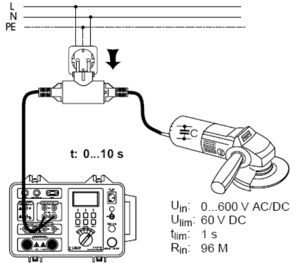
图 22. 检测线的连接
