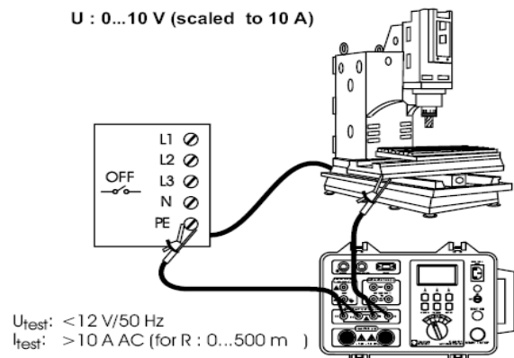
图 11. 检测线的连接
