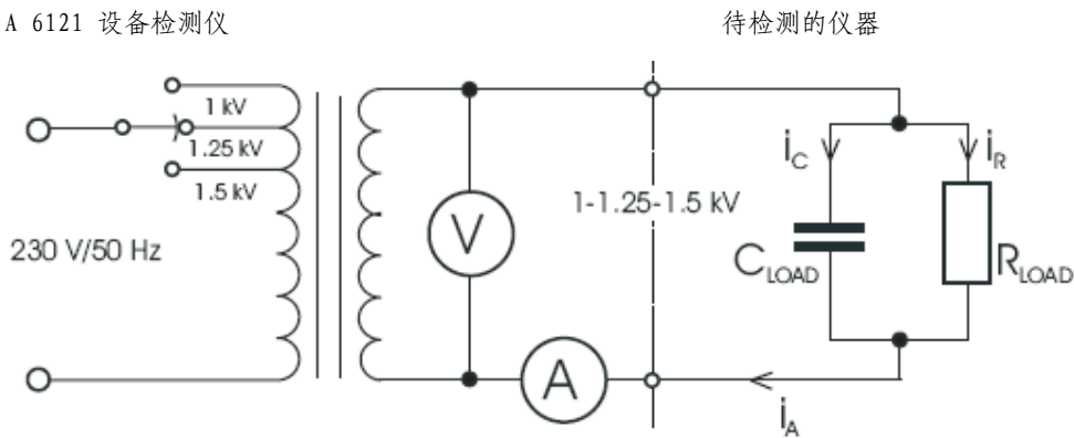
图 2. 检测电流
