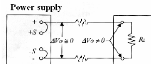
图 6-2 电源供应器的局部误差侦测
