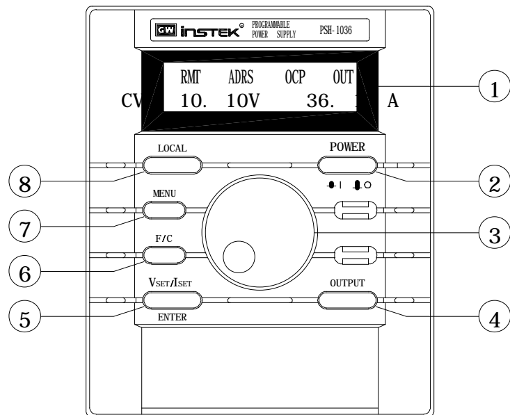
前面板图
