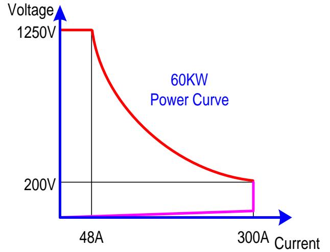
36360E 功率曲线图
