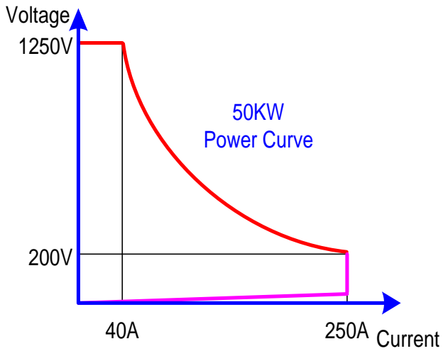
36350E 功率曲线图
