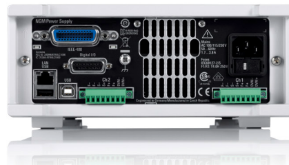
R&amp;S®NGM202, 后视图
