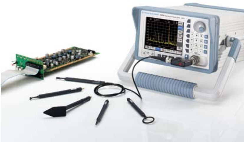
R&S®HZ-15 近场探头组、台式频谱分析仪和R&S®HZ-16外置预放大器
