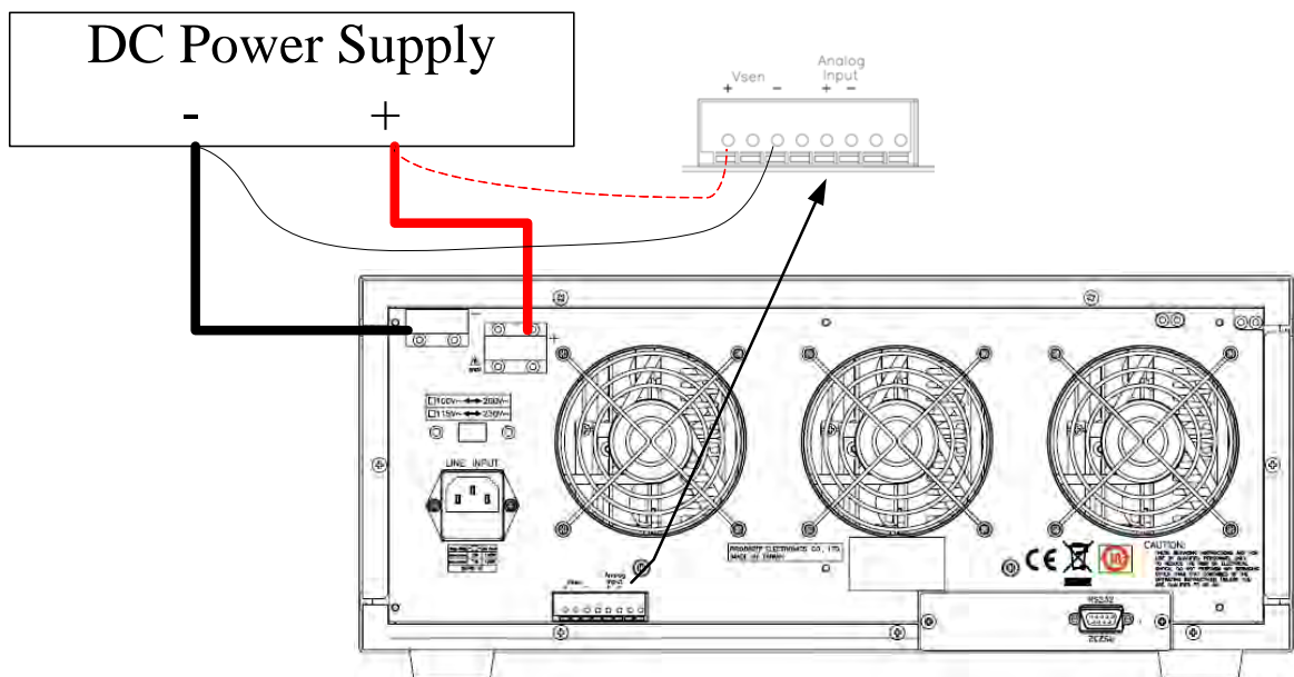
圖 5-2 遠地電壓檢知連接圖
