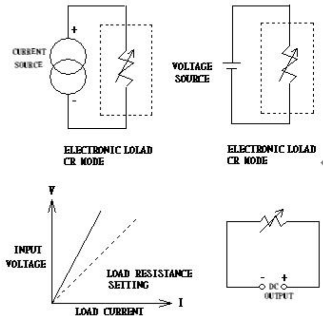
圖 5-6 固定電阻操作模式之應用
