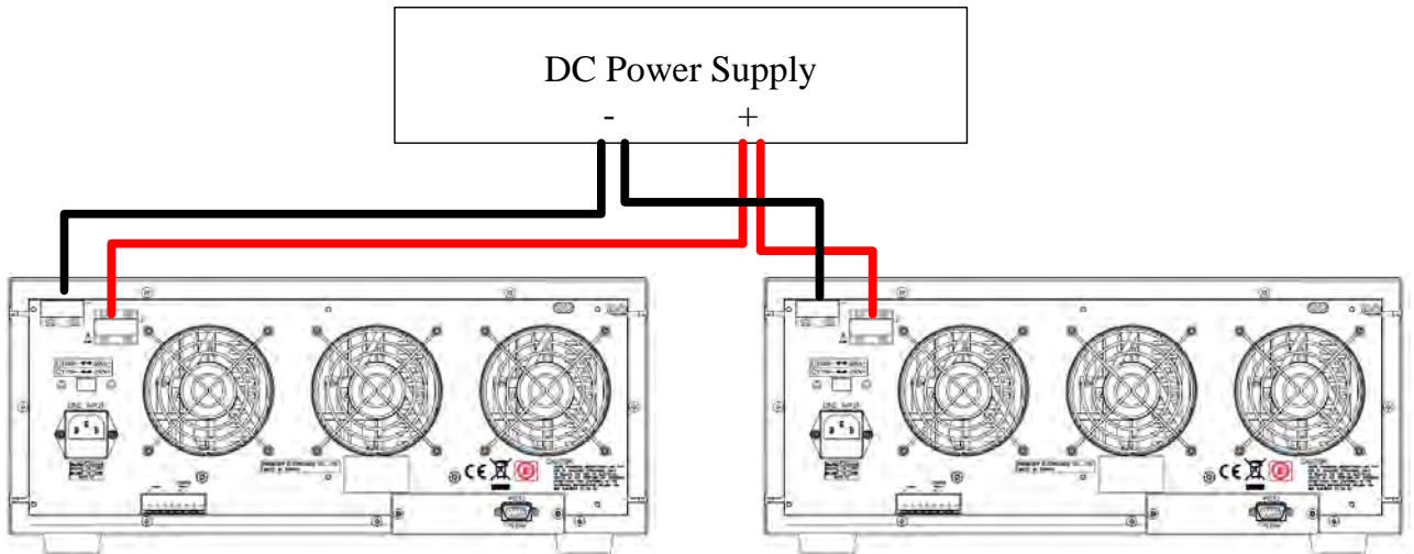
圖 5-10 電子負載多組並聯之連接圖
