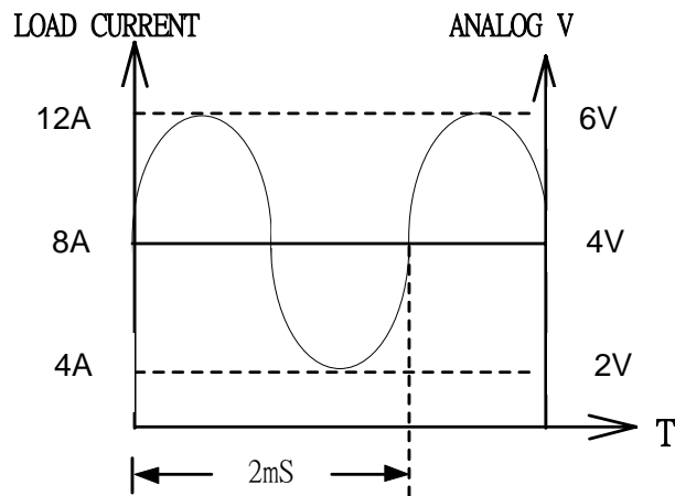
圖 3-4 負載電流之類比設定輸入
