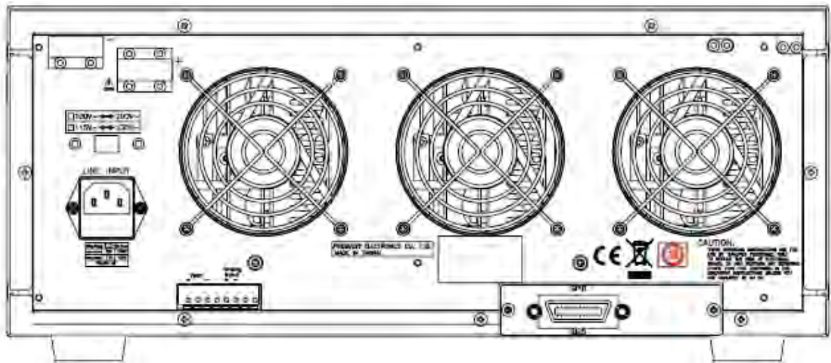
圖 2-3 3360F 系列GPIB連接埠
