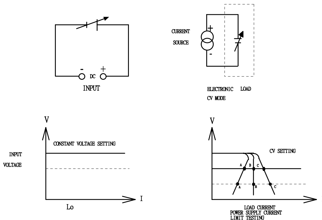
圖 5-5 固定電壓操作模式之應用
