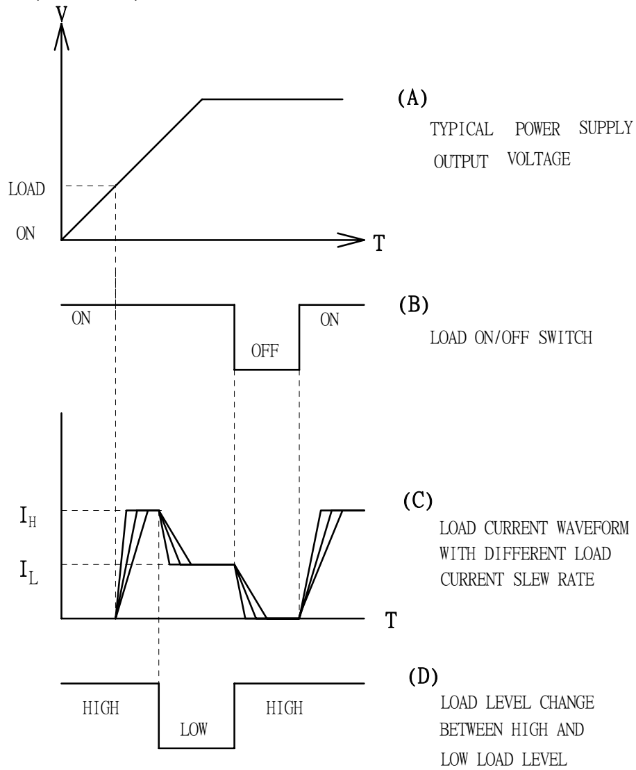
圖 2-7 負載電流波形與 LOAD ON/OFF 開關，負載準位與電源供應器之輸出電壓間的關係圖
