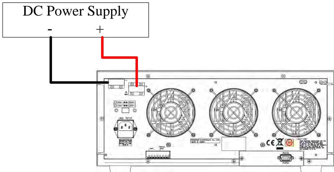
圖 5-1 本地電壓檢知連接圖
