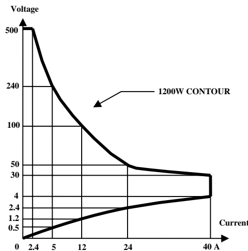
圖 1-2 3361F 高功率電子負載功率曲線圖
