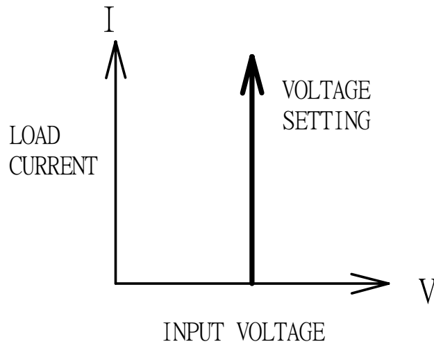
圖 1-7 固定電壓模式特性圖
