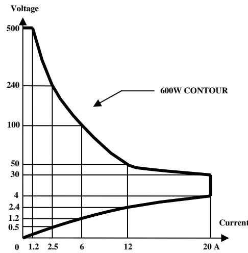
圖 1-1 3360F 高功率電子負載功率曲線圖
